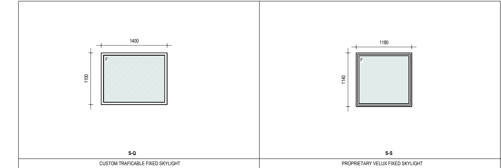
SKYLIGHT LEGEND 1 : 50
